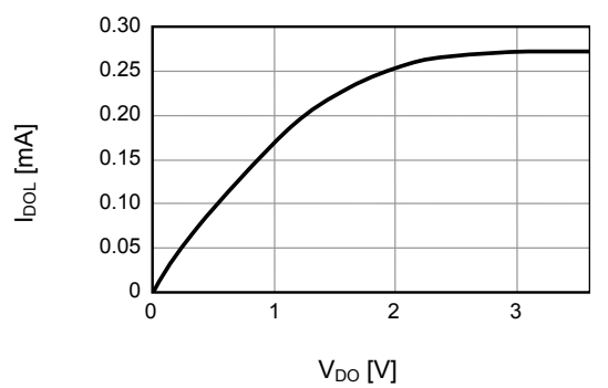
4. I_{DOL} - V_{DO}
