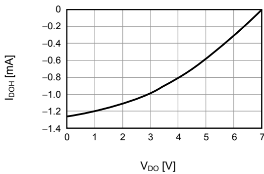
3. I_{DOH} - V_{DO}
