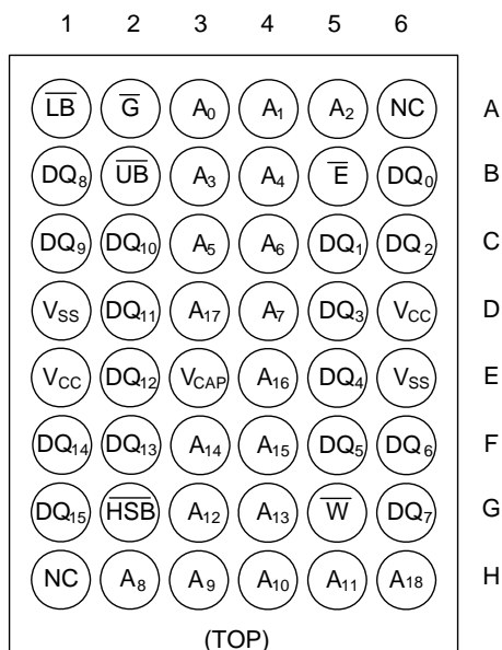
48-Ball FBGA
