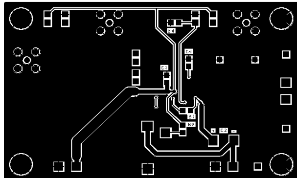
Bottom Layer
