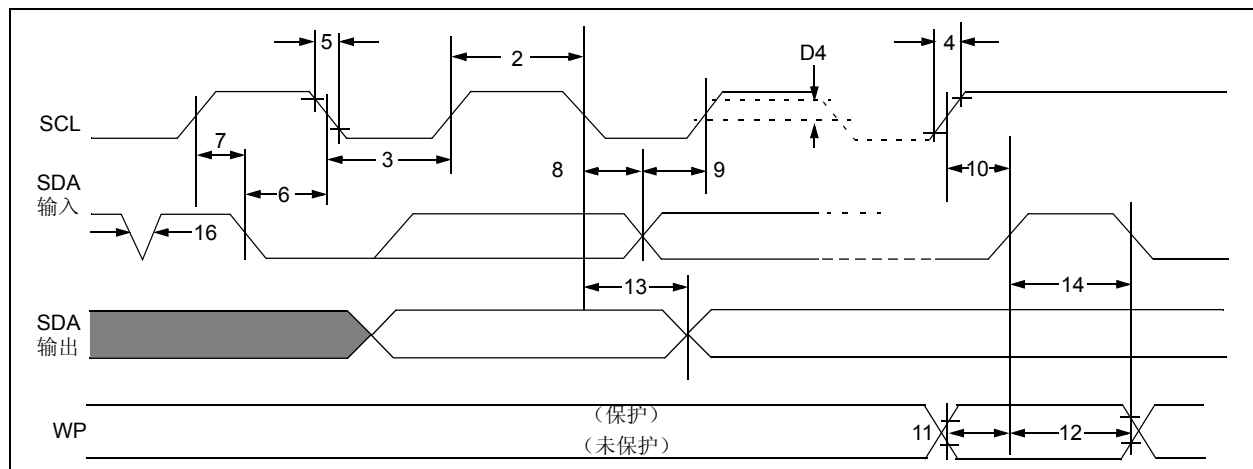
图 2-1: 总线时序
