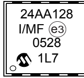
8 引脚 5x6mm DFN 封装标识（无铅）
