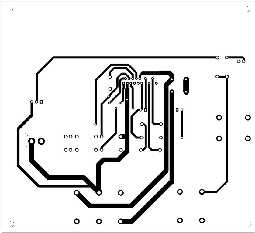
Bottom Layer
