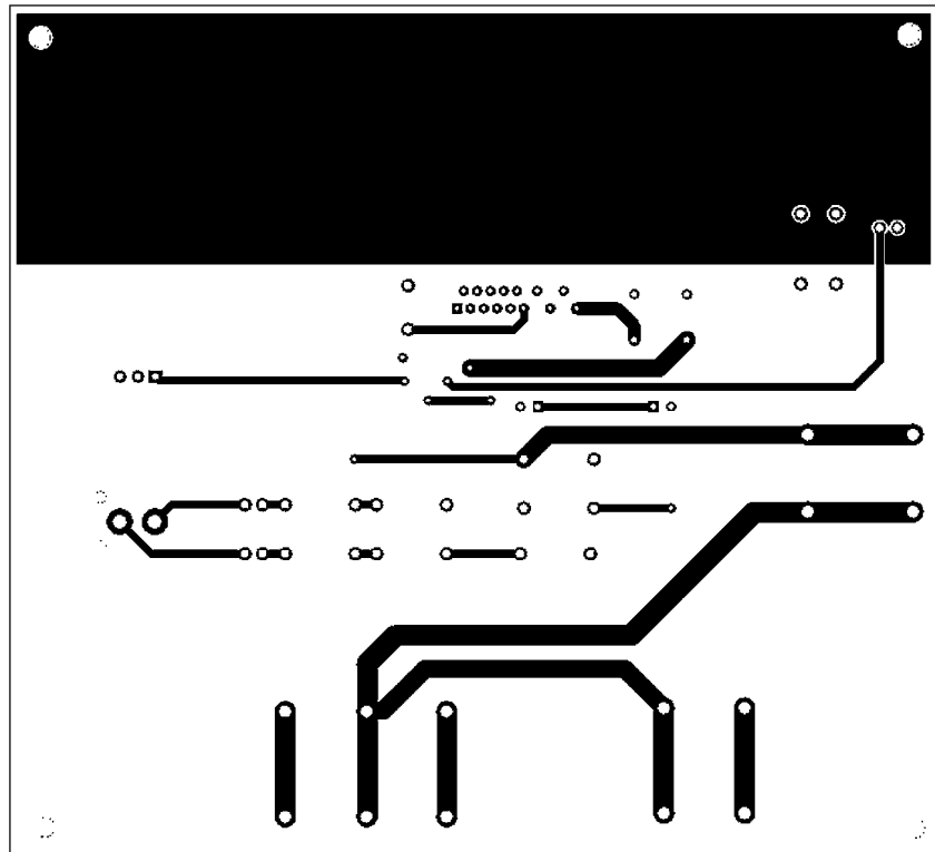
Top Layer
