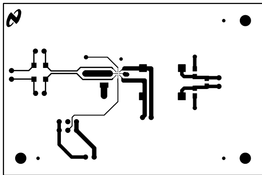
Top Layer
