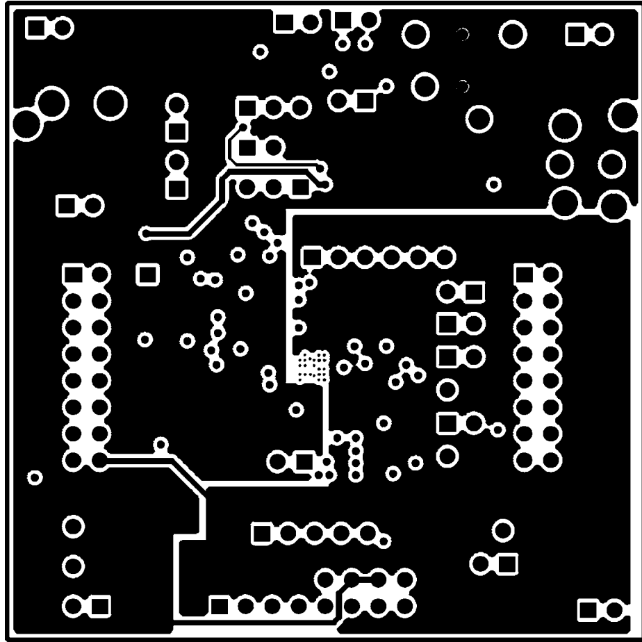
Mid Layer 1
