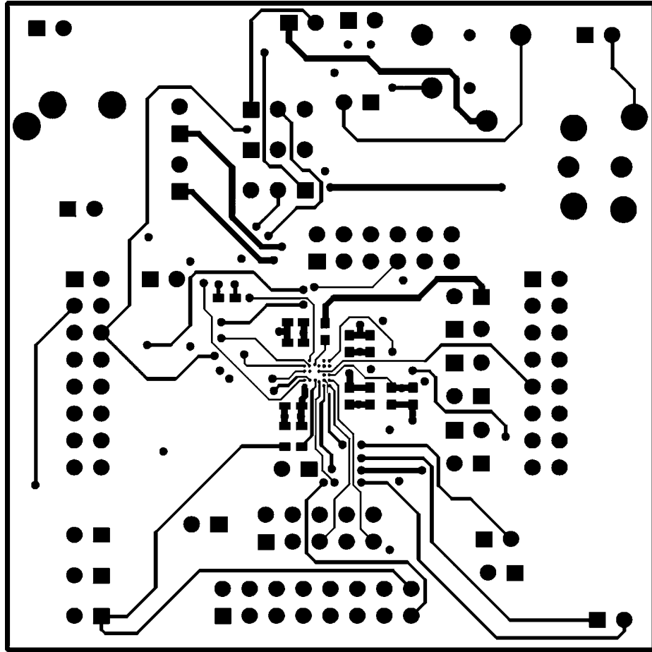
Bottom Layer
