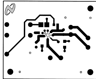
Top Layer
