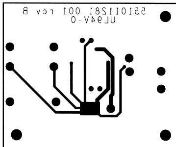
Bottom Layer
