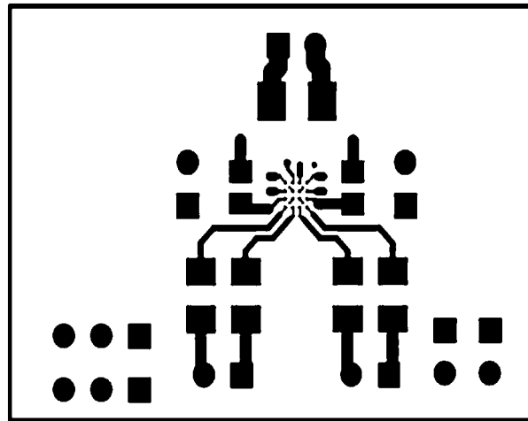
Top Layer
