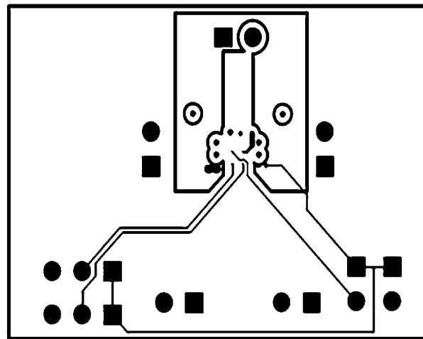
Mid 1 Layer
