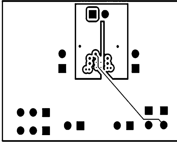
Mid 2 Layer
