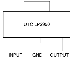
SOT-252 Package
