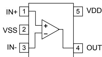
SSOP5
