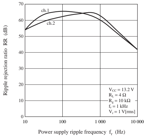
RR — f_r
