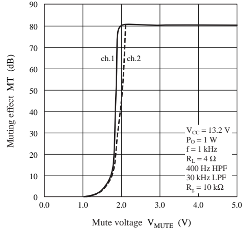
MT — V_{MUTE}
