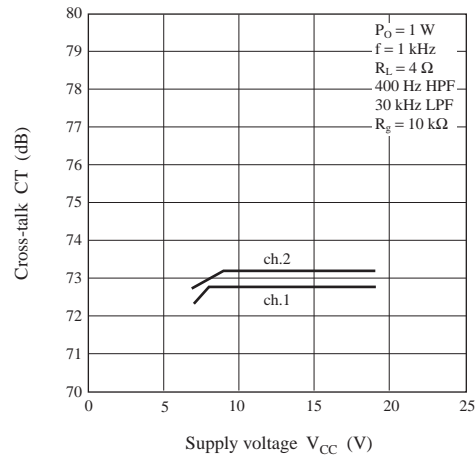
CT — V_{CC}
