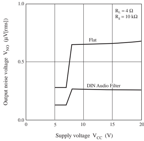
V_{NO} - V_{CC}
