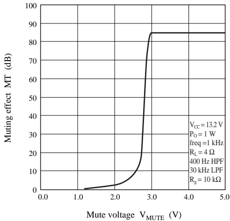
MT — V_{MUTE}
