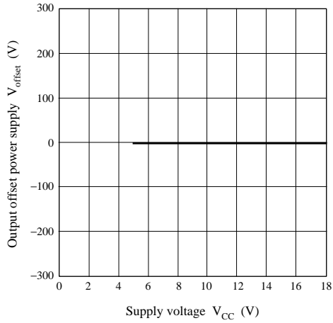
V_{OFFSET} — V_{CC}
