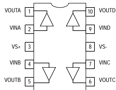
EL 5421C (MSOP 10)
