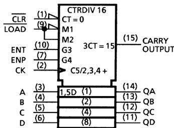
TC74ACT161
