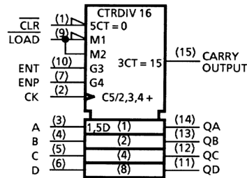
TC74ACT163
