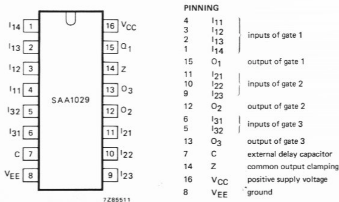
Fig. 2 Pinning diagram.
