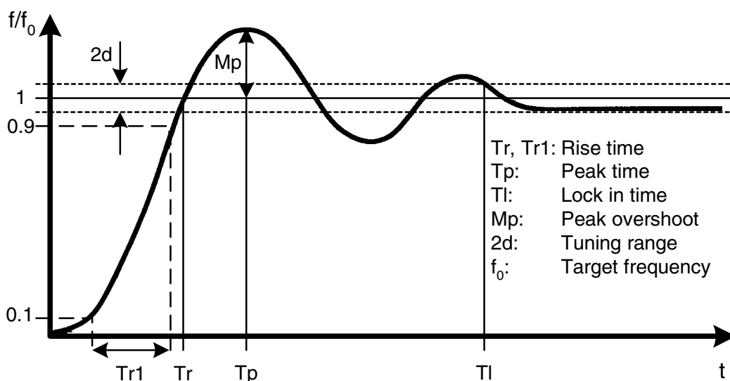
Figure 20 Transient Parameters
