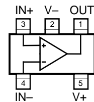
SOT-23-5 (M5)
