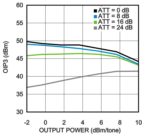
OIP3 vs. Pout
