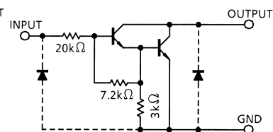
TD62105P / F
