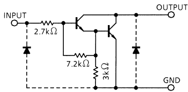
TD62103P / F
