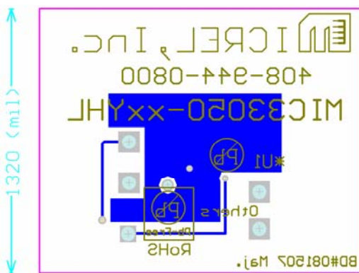
Bottom Layer
