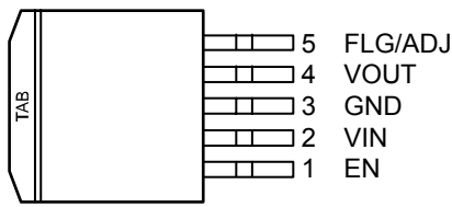
S-PAK-5 (R) TO-263-5 (U)
