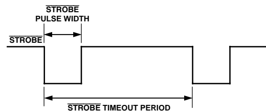
Figure 4. \overline{\text{STROBE}} Parameters
