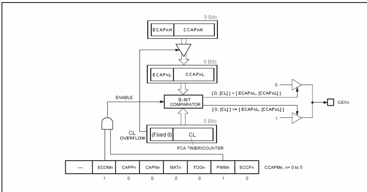
Figure 14-7. PCA PWM Mode
