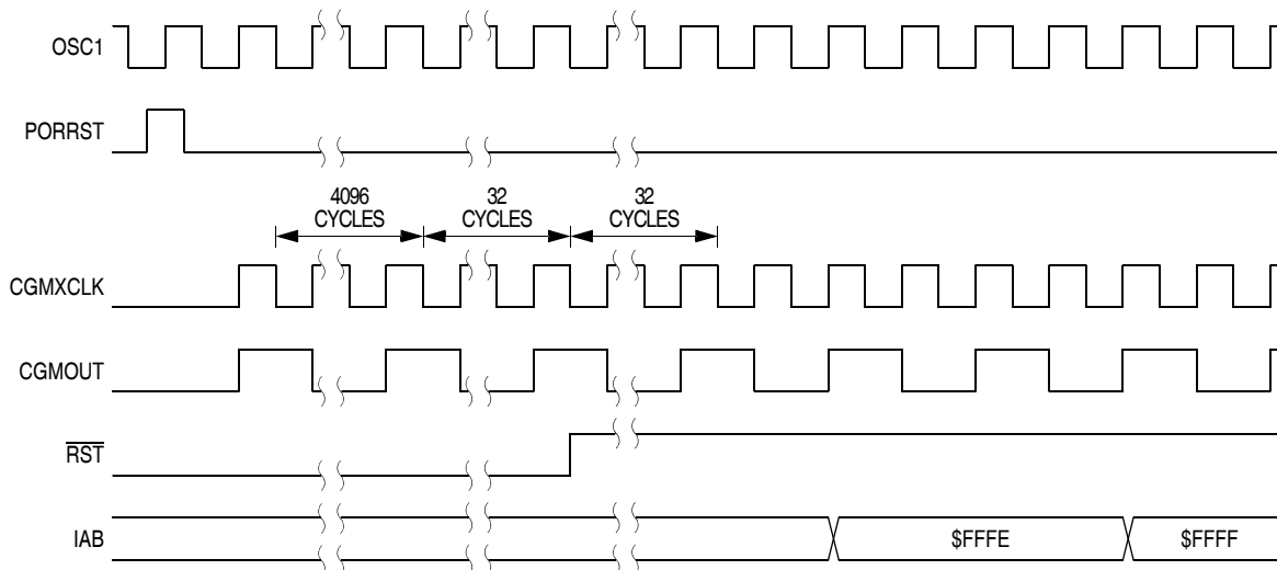
Figure 7-6. POR Recovery
