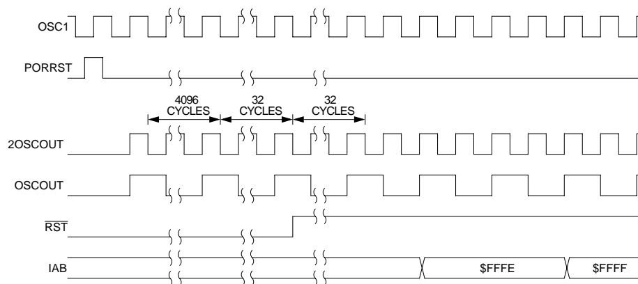
Figure 7-7. POR Recovery
