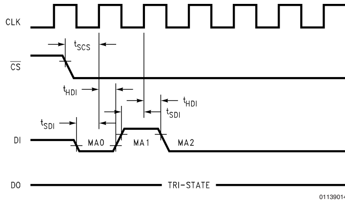
FIGURE 3. DI Timing
