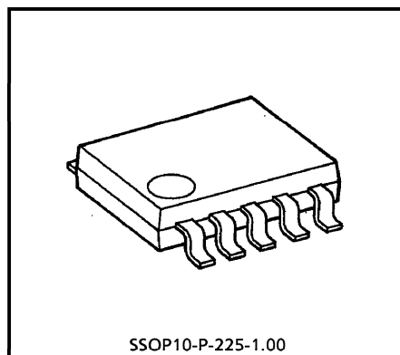
SSOP10-P-225-1.00
