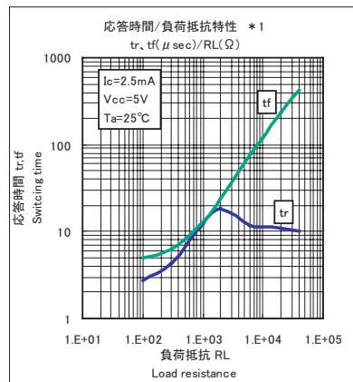
*1応答時間特性図
