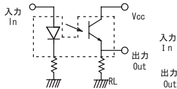
*1応答時間特性図
