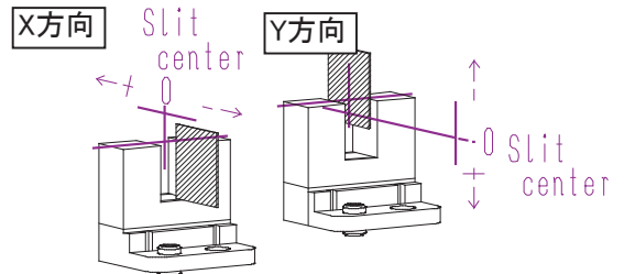
*2 位置検出特性図
