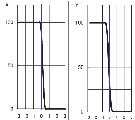
*2 位置検出特性図
