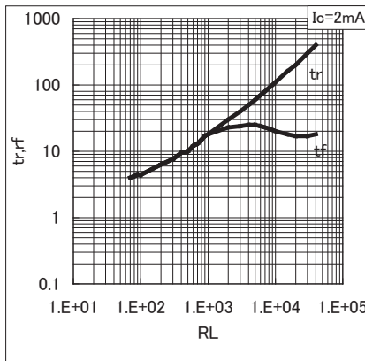
*1応答時間特性図
