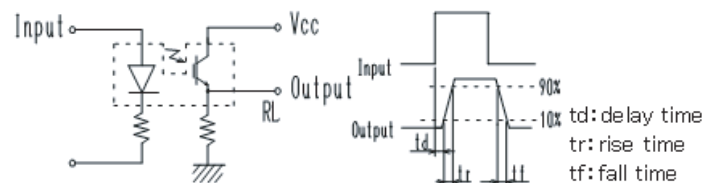
*1 応答時間特性
