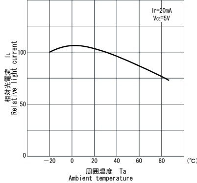
■相対光電流/周囲温度特性 I_L/T_a
