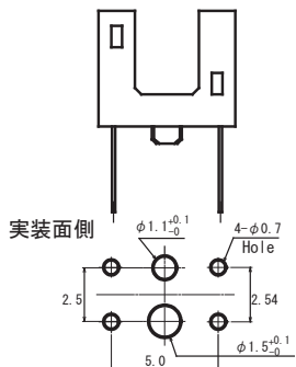
推奨取付穴寸法
