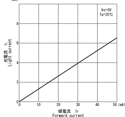
■光電流/順電流特性 I_L/I_F
