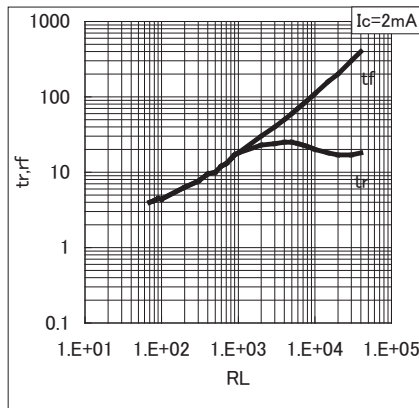
*1応答時間特性図
