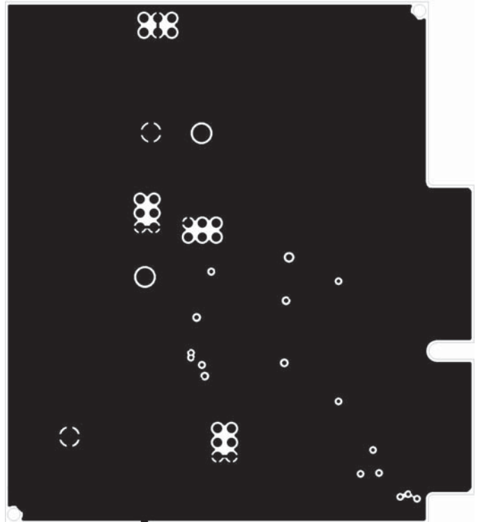
Layer 4 GND
