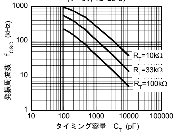
発振周波数対タイミング容量特性例
