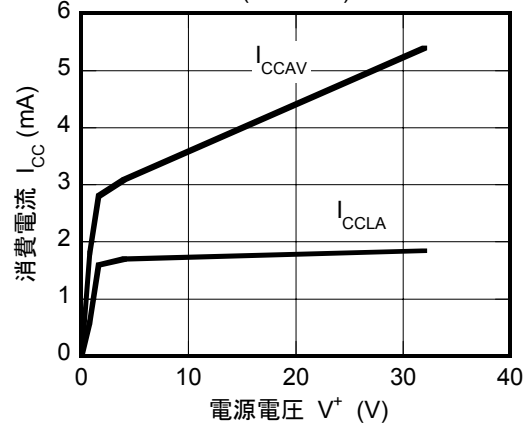
消費電流対電源電圧特性例
