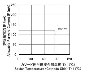
■ カソード側半田接合部温度-許容順電流特性 Solder Temperature (Cathode Side) vs. Allowable Forward Current
