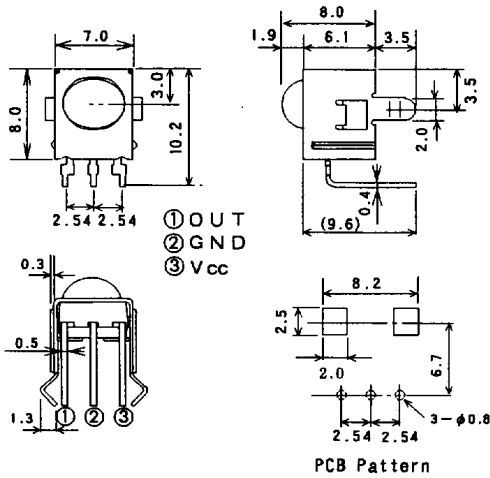
NJL62H000A UNIT : mm
