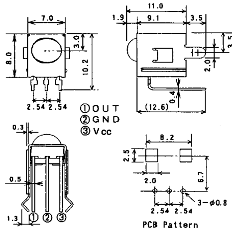
NJL63H000A UNIT : mm
