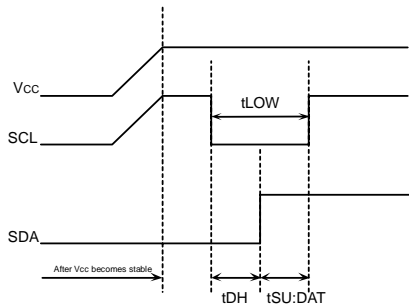
Fig.57 When SCL='H' and SDA='L'
