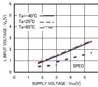
Fig.4 'L' input voltage V_{IL} (A0,A1,A2,SCL,SDA,WP)
