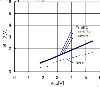
Fig.4 L input voltage VIL,2 (SCL.SDA,WP)
