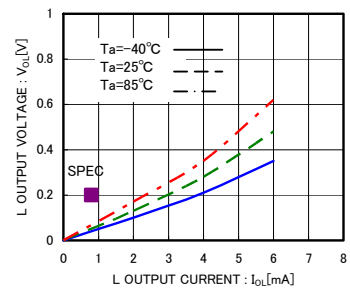
Fig.5 'L' output voltage V_{OL-I_{OL}} ( V_{CC}=1.7V )
