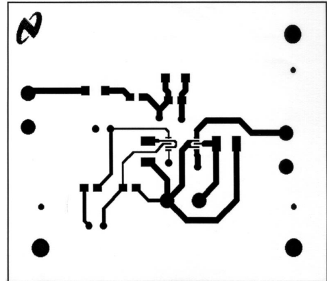
Top Layer
