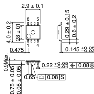
MSOP8
