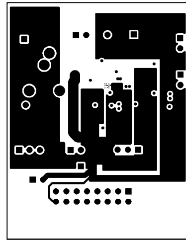
Internal Layer 1
