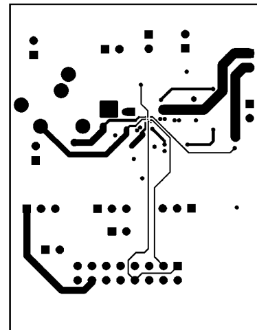
Bottom Layer
