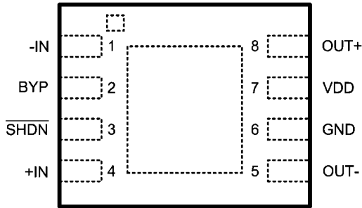
LLP Package
