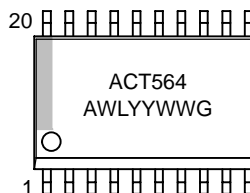
SOIC–20W
