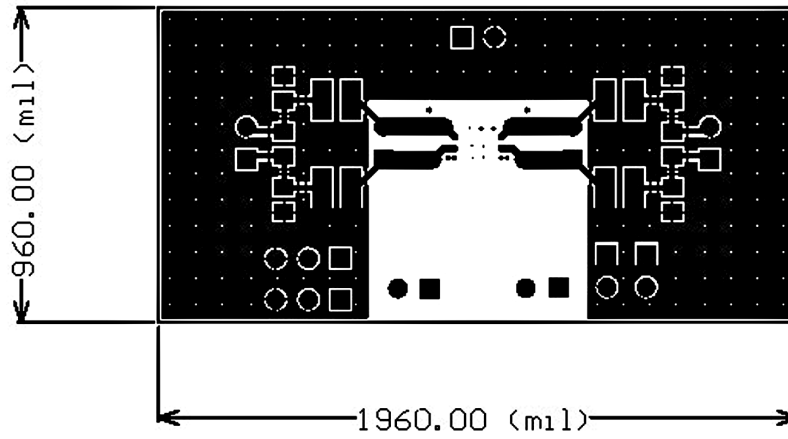
Layer 4
