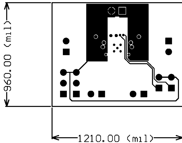
Layer 2
