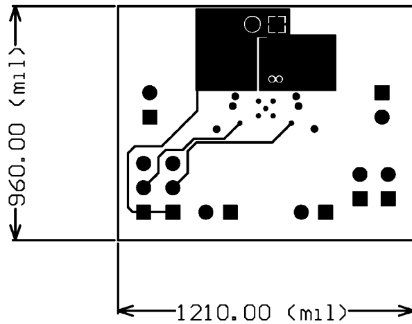
Layer 3
