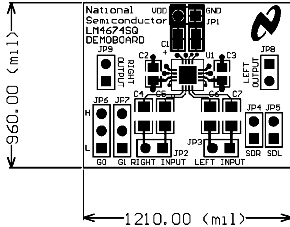
Layer 1
