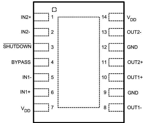
LLP Package
