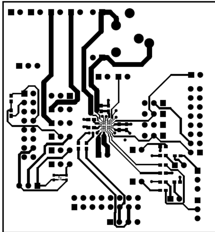
FIGURE 26. Top Layer
