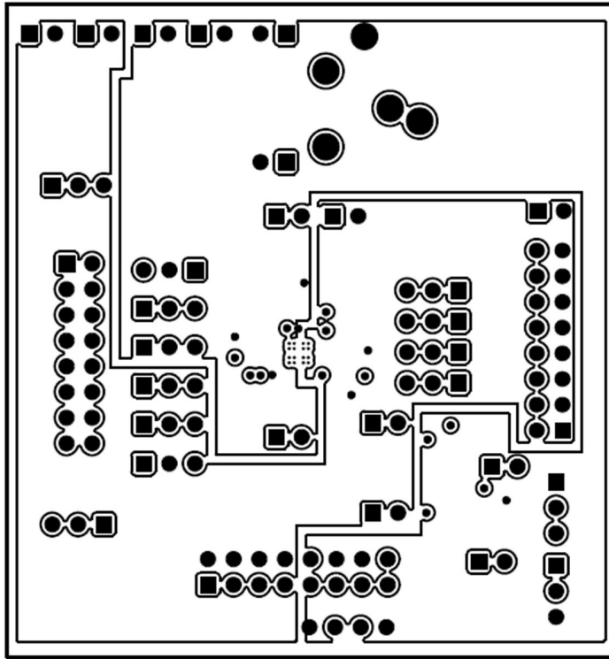
FIGURE 27. Inner Layer 1
