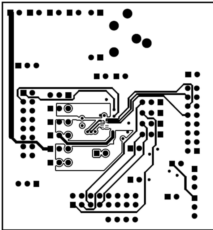
FIGURE 28. Inner Layer 2
