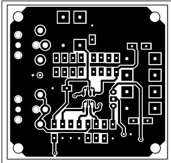
Fig. 106 : SO8 & MiniSO8 Demoboard Bottom Solder Layer
