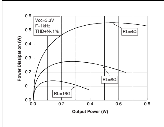
Fig. 23 : Power Dissipation vs Pout
