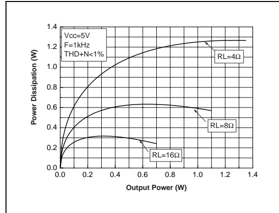
Fig. 22 : Power Dissipation vs Pout
